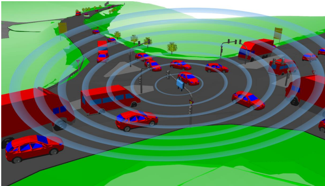
Abbildung 36: Schema aus der Funkplanung für RoadSideUnits (RSU) z.B. an Kreuzungen.
