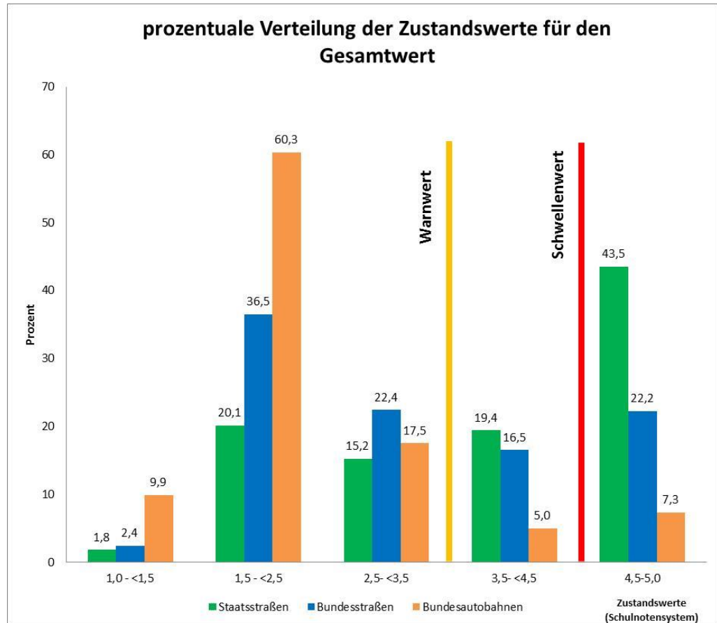
Abbildung 4: Zustand der Staats-, Bundesstraßen und Bundesautobahnen im Freistaat Sachsen
